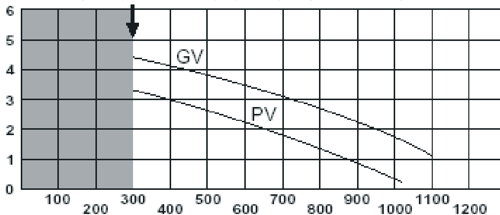
Graf závislosti výtlačku čerpadla v metrech vod. slp. na průtoku topné vody (termostatické ventily uzavřené).
