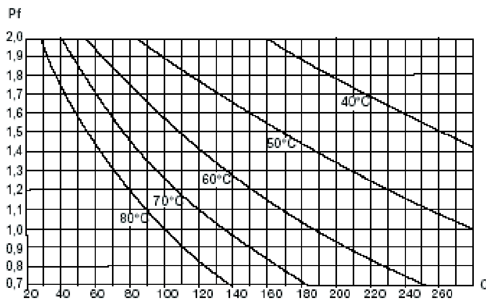
Graf použití expanzní nádoby
