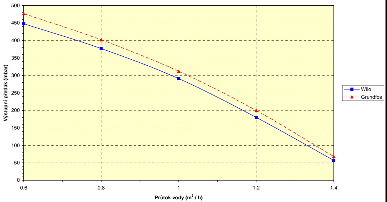
Připojovací přetlak THERM 20 a 28 CXE
