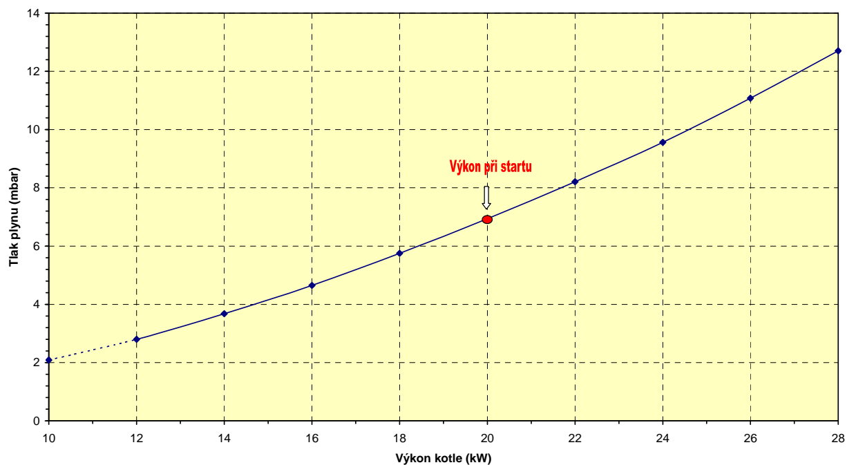
Graf nastavení výkonu THERM 28 CXE, LXE, LXZE (zemní plyn), trysky - 0.82 mm
