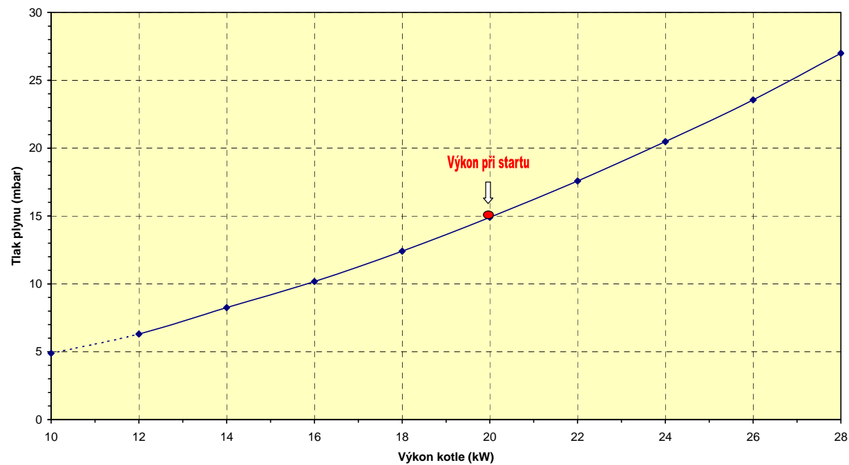
Graf nastavení výkonu THERM 28 CXE, LXE LXZE (propan), trysky - 0.51 mm
