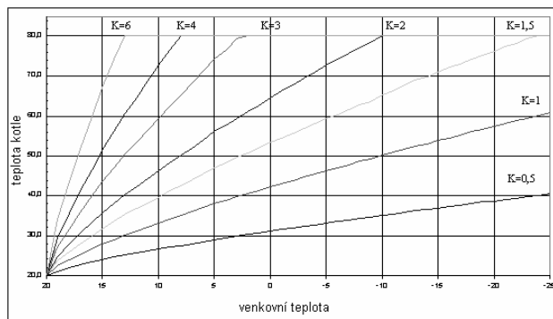
Sklony ekvitermy
