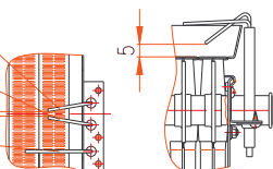
Detail elektrod
