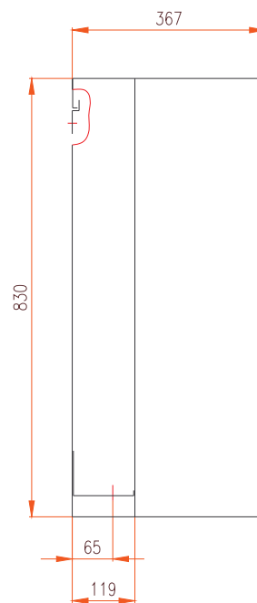
ŘEZ II-II
