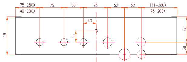
Detail elektrod
