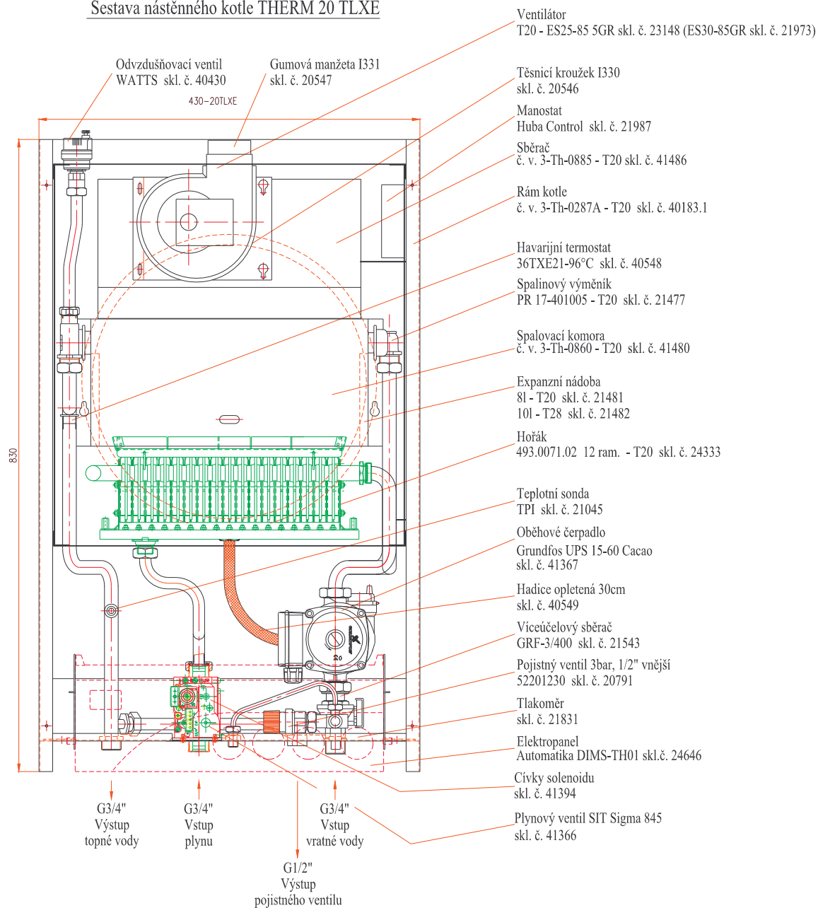
Sestava nástěnného kotle THERM 20 TLXE
