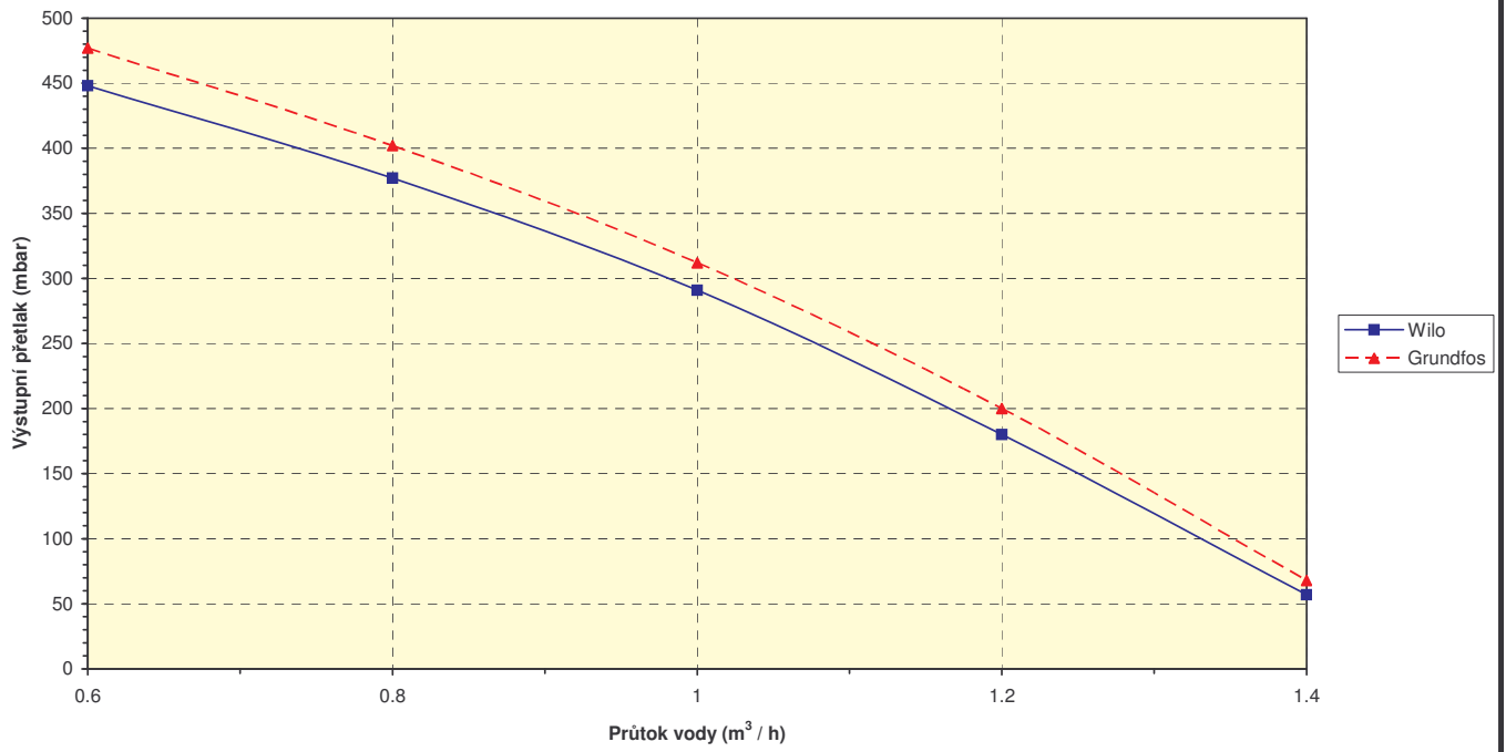
Připojovací přetlak THERM 20 TCXE
