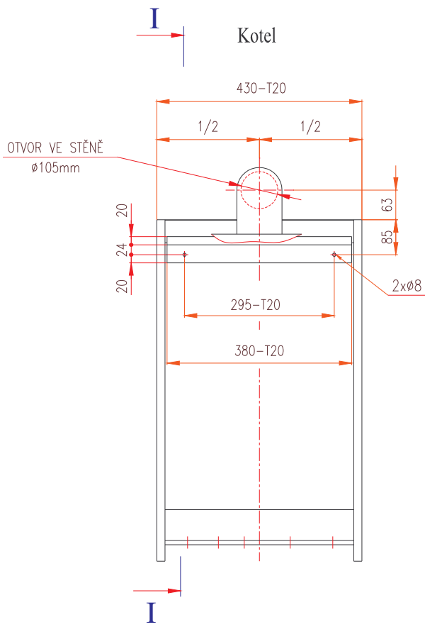
ŘEZ I-I
