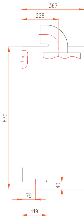
ŘEZ I-I
