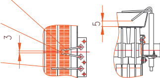
Detail elektrod
